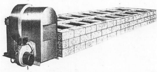
รูปที่ 1 เครื่องลดความชื้นแบบข้าวเปลือกบรรจุในกระสอบ[1]
