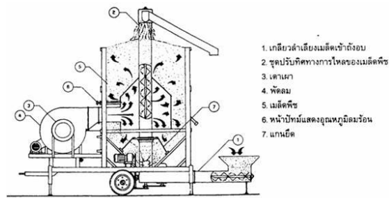
รูปที่ 3 เครื่องลดความชื้นข้าวเปลือกแบบถังหมุนเวียน [1]
