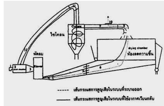
รูปที่ 8 เครื่องลดความชื้นข้าวเปลือกแบบฟลูอิดไดซ์เบด [3]
