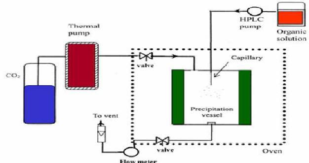
รูปที่ 6 รูปแบบและหลักการเครื่องมือแบบ Supercritical antisolvent (SAS) 22
