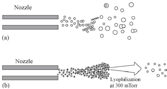
รูปที่ 3 แผนผังของเทคนิค (a) Rapid expansion of supercritical solution (RESS) และ (b) Supercritical solution with solid cosolvent (RESS-SC) (ในที่นี้ + คืออนุภาคของเมนทอลและ o คืออนุภาคของสาร) 17,18
