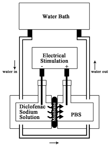
รูปที่ 1 ส่วนประกอบและระบบการทำงานของ Franz diffusion cell ในการศึกษาวิจัยถึงความสามารถในการซึมผ่านของยา
