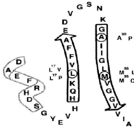
รูปที่ 4 โครงสร้างทุติยภูมิของ Aβ แสดงลำดับกรดอะมิโนของสายเปปไทด์ Aβ 1-42 และการเกิดโครงสร้างทุติยภูมิโดยอยู่ในรูปแบบสาย alpha helix 1 สายซึ่งมีลักษณะเป็นเกลียวขดคล้ายสปริง และ beta sheet 2 สาย โดยกรดอะมิโนที่ถูกระบุแสดงถึงการถูกแทนที่ด้วยกรดอะมิโนตัวอื่น 49
