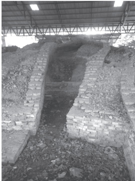
ภาพแสดงที่ 7 ส่วนรายละเอียดด้านหน้าของเตาเผา
