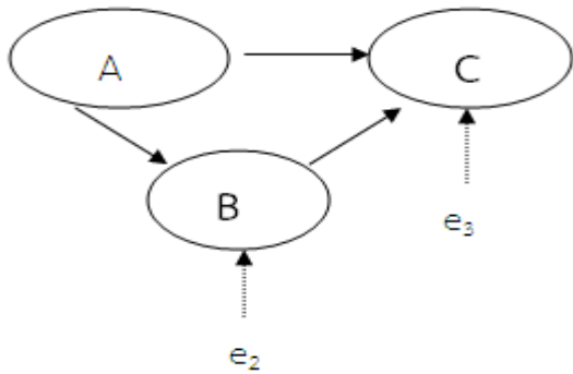
ภาพ 1 โมเดลแบบทิศทางเดียว (Recursive Model)
