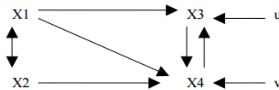
ภาพ 7 โมเดลที่เกิดปัญหา Under-estimate
