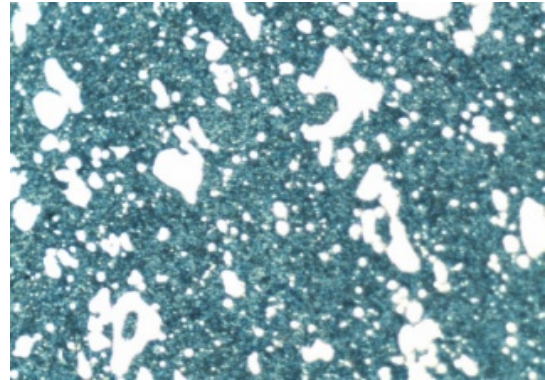
รูปที่ 7 โครงสร้างเหล็กกล้าเครื่องมือ JIS SKD 11 ที่ผ่านกระบวนการอบชุบทางความเย็นอุณหภูมิ -80°C
