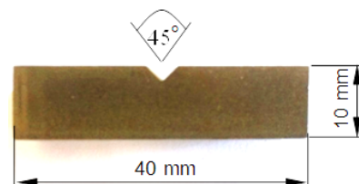
รูปที่ 3 ชิ้นทดสอบแรงกระแทก
