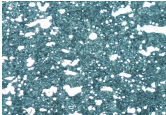
รูปที่ 6 โครงสร้างเหล็กกล้าเครื่องมือ JIS SKD11 ที่ผ่านกระบวนการอบชุบทางความเย็นอุณหภูมิ -20°C
