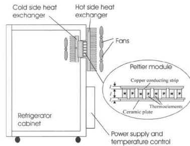
ภาพที่ 1 โครงสร้างของตู้เย็นด้วยเทอร์โมอิเล็กทริก
