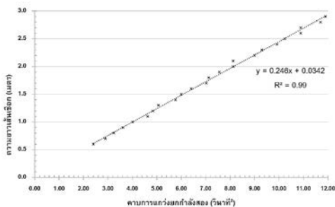
ภาพที่ 8 กราฟความสัมพันธ์ระหว่างความยาวเส้นเชือกและคาบการแกว่งยกกำลังสอง
