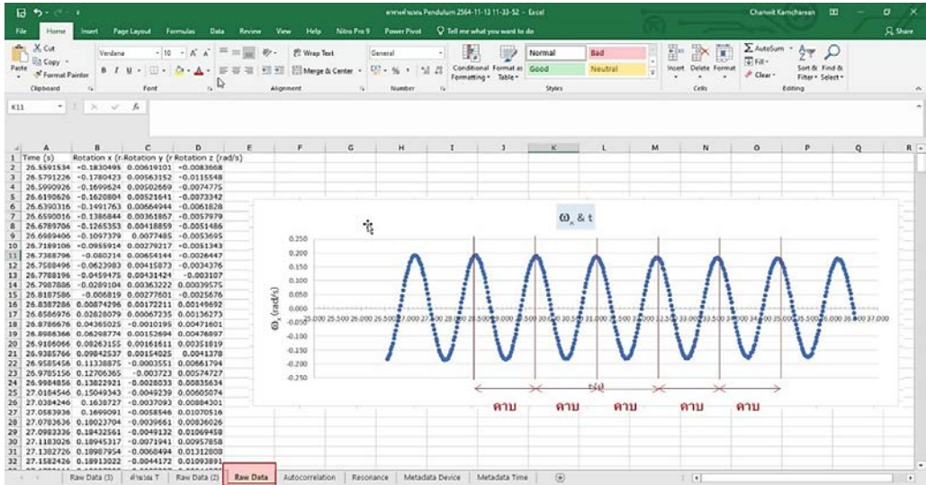
ภาพที่ 6 คาบการแกว่งของสมาร์ตโฟน
